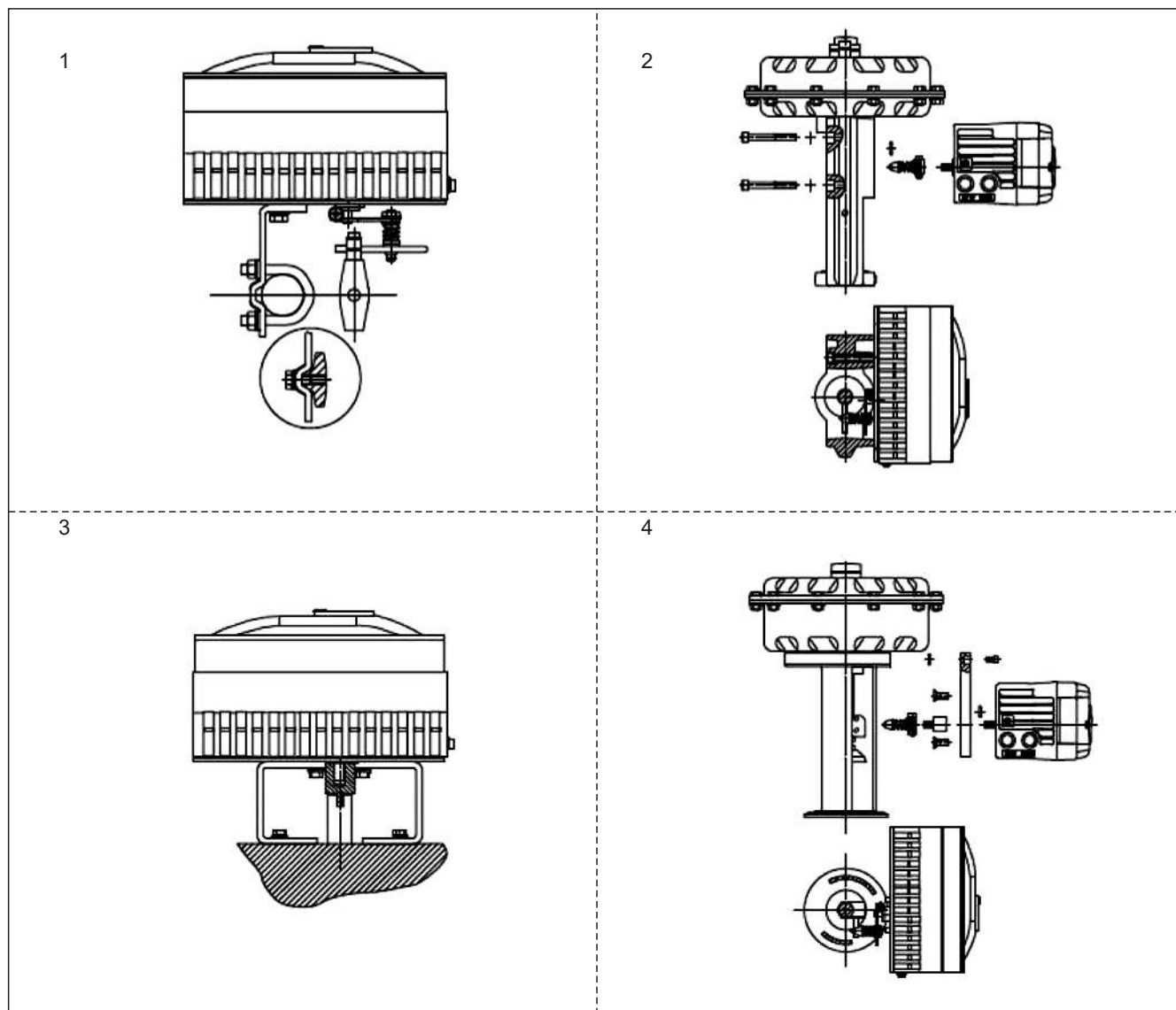
图43 不同的安装方式
