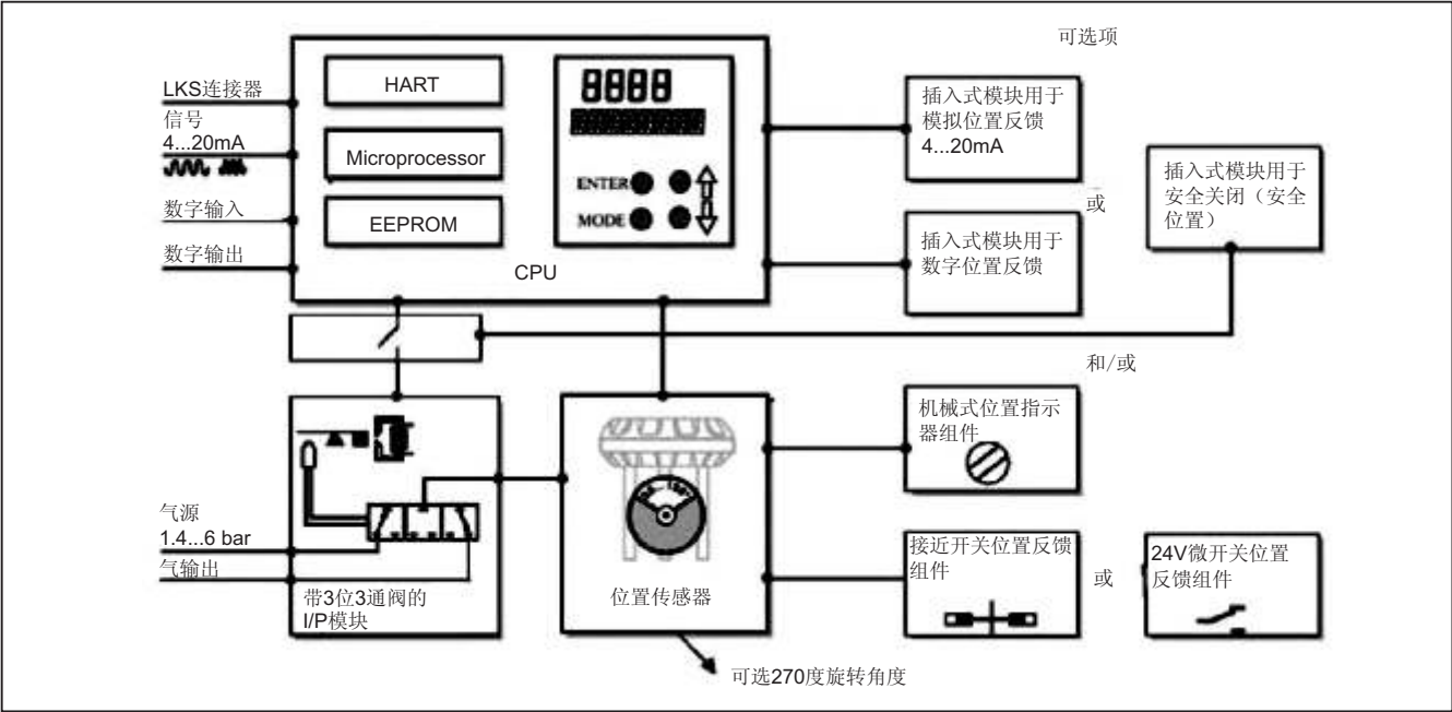
图1: TZIDC原理图
