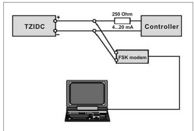
图6：通过信号线用FSK modem进行HART通信
