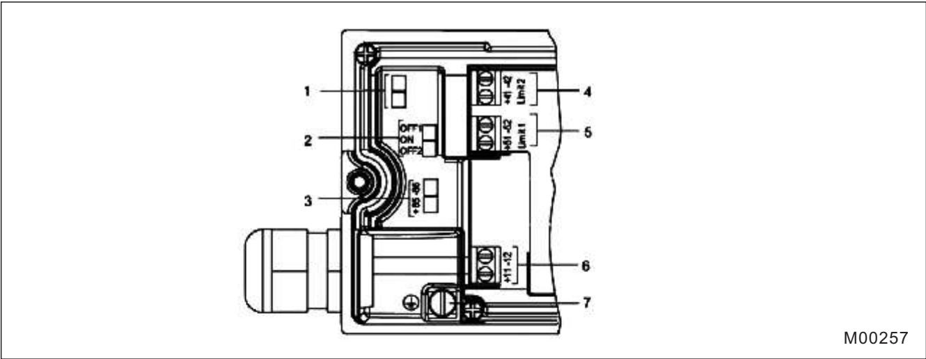
图21 端子分布图
