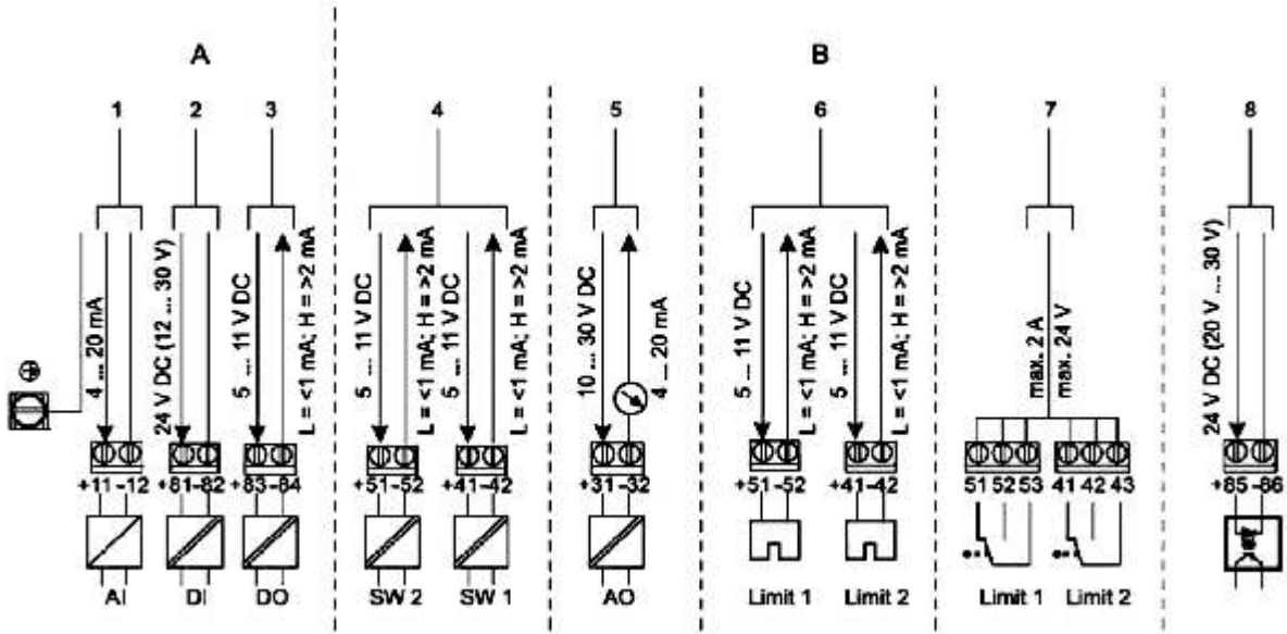
图7 端子分布图
