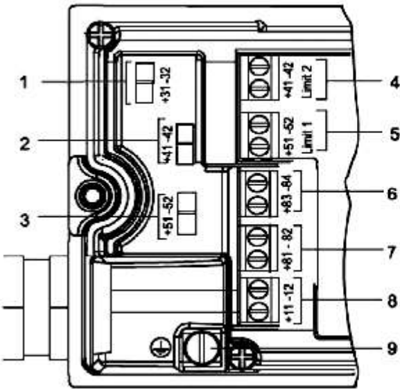
图7 端子分布图
