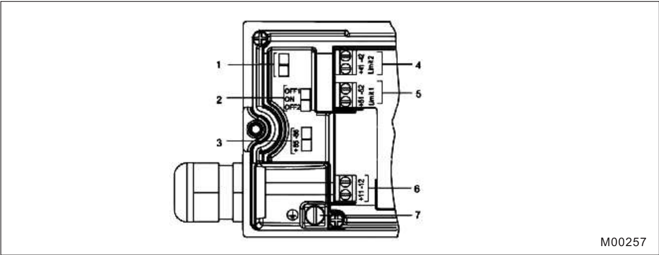
图31 端子分布图
