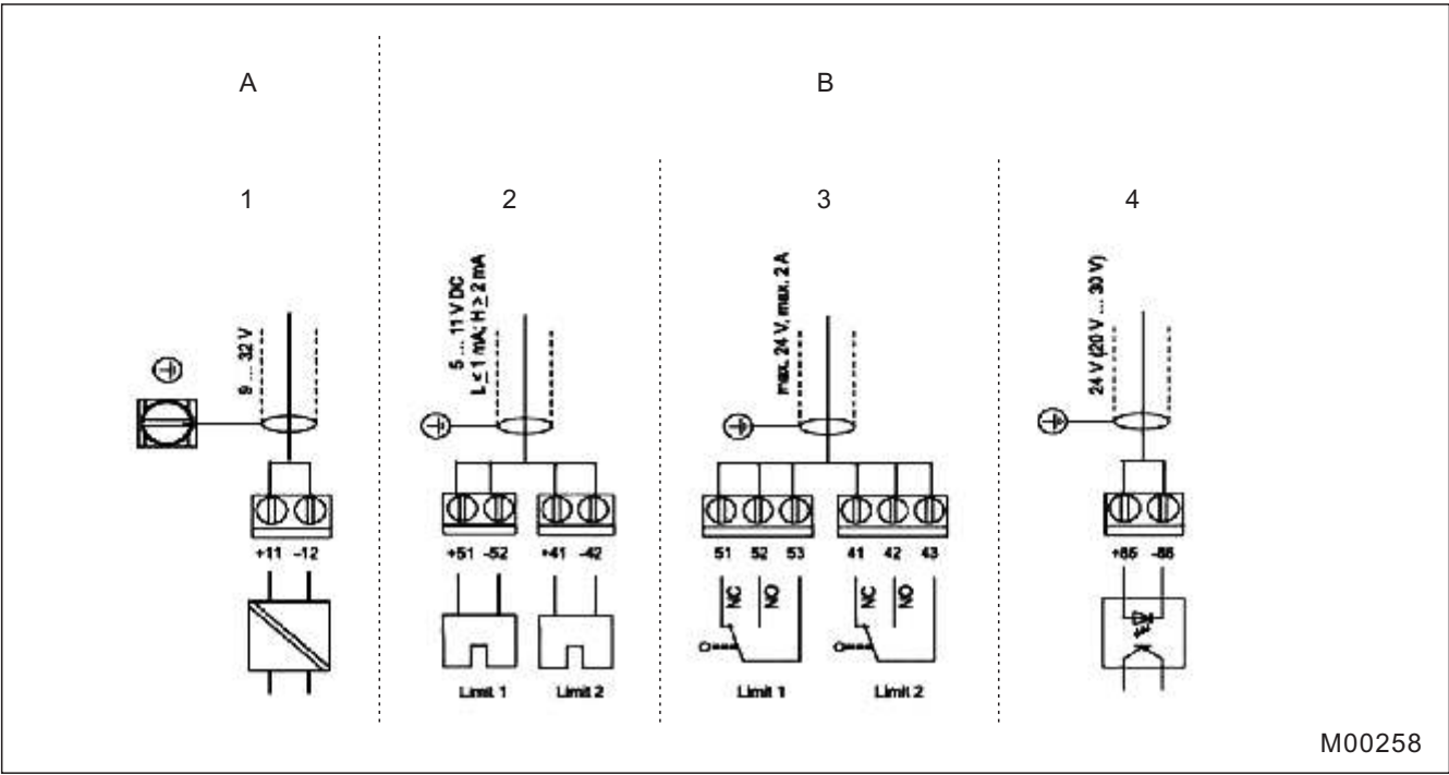
图22 接线配置图
