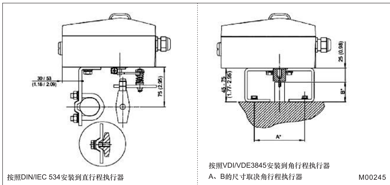
图12 安装图
