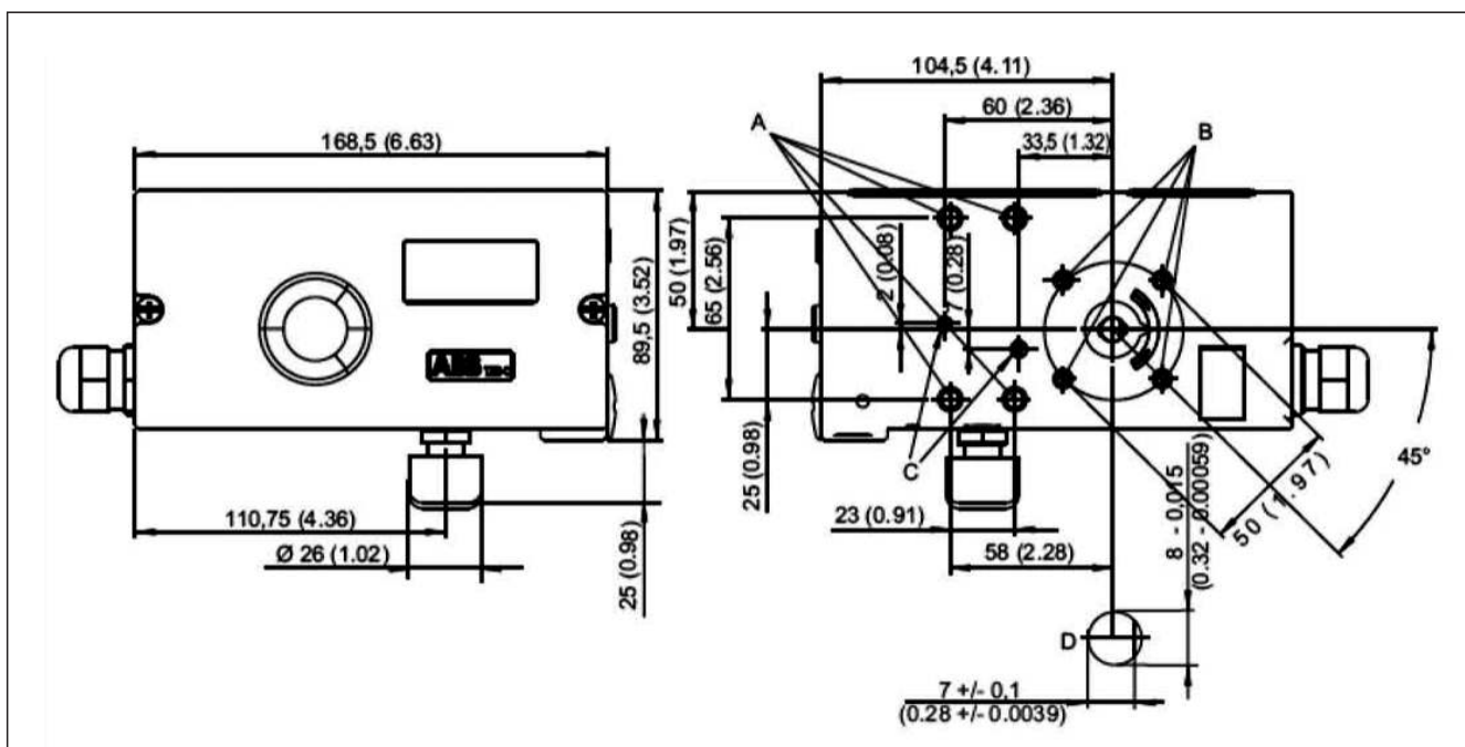
图10 前视图和后视图
