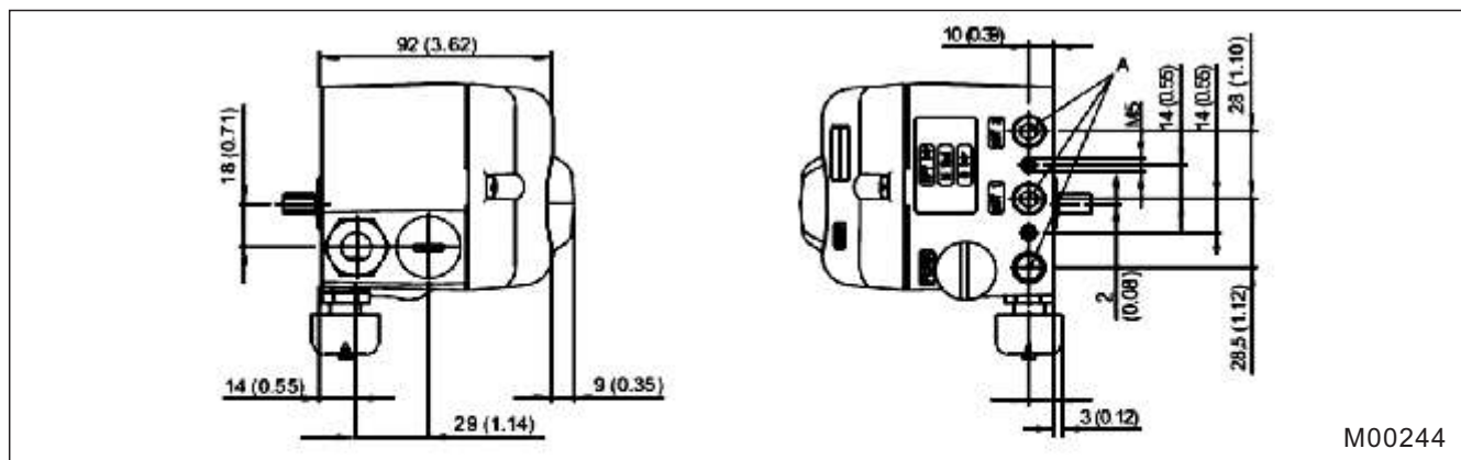
图11 侧视图（从左到右）
