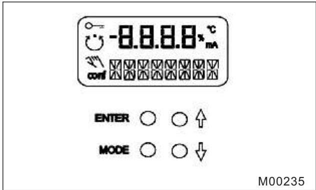
图4 TZIDC的操作按键和显示屏
