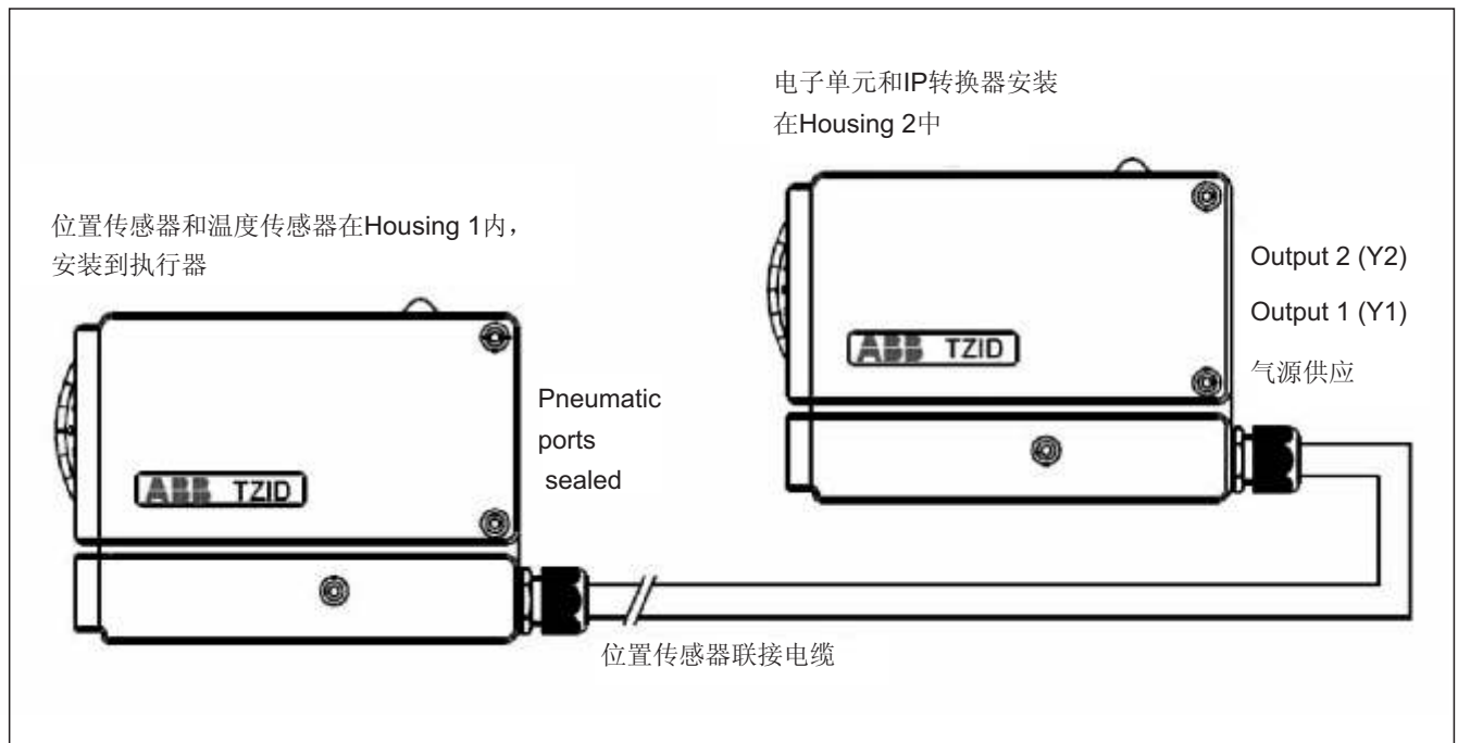
图50 分体式定位器的示意图
