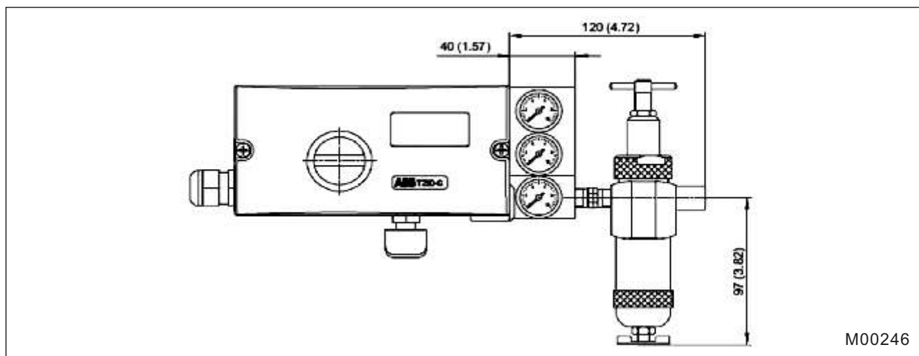
图13 带压力表组件和减压过滤器的TZIDC定位器
