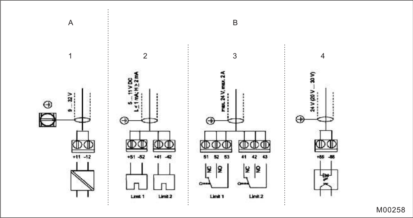
图32 接线配置图
