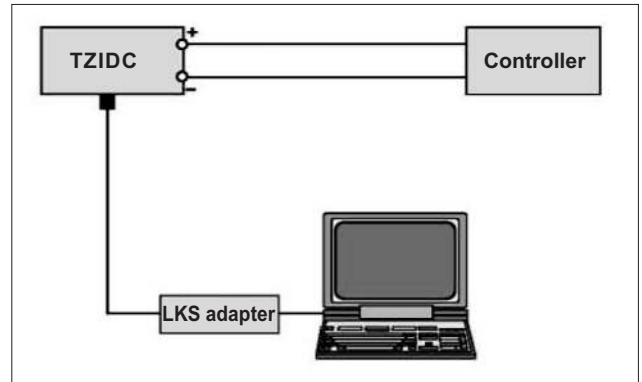
图5：通过LKS适配器进行本地通信
