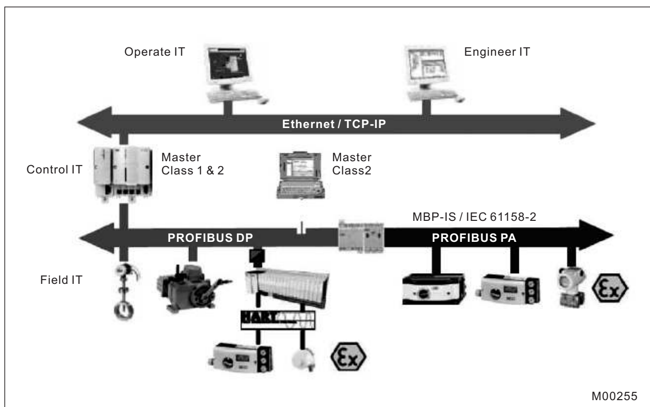
图20 以PROFIBUS协议进行通讯
