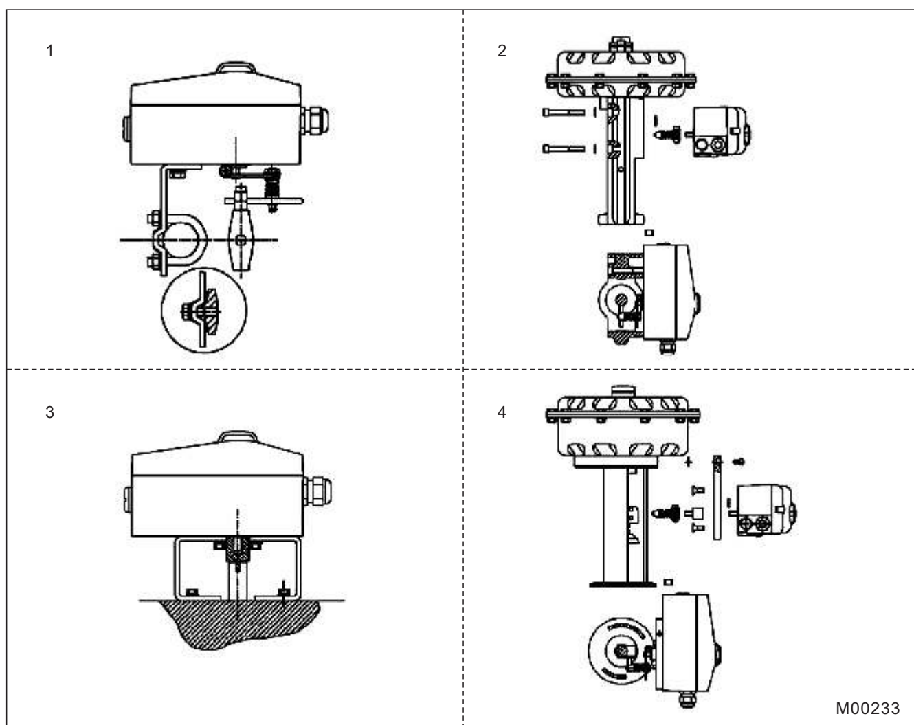
图2 不同的安装方式
